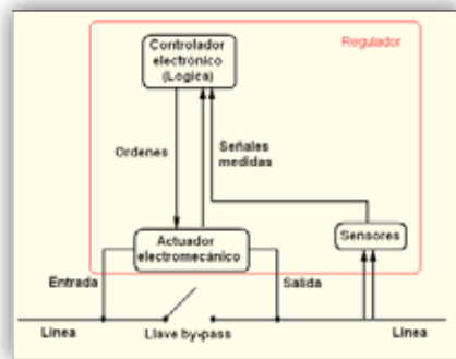
Esquema de bloques funcionales de un regulador de tensión
